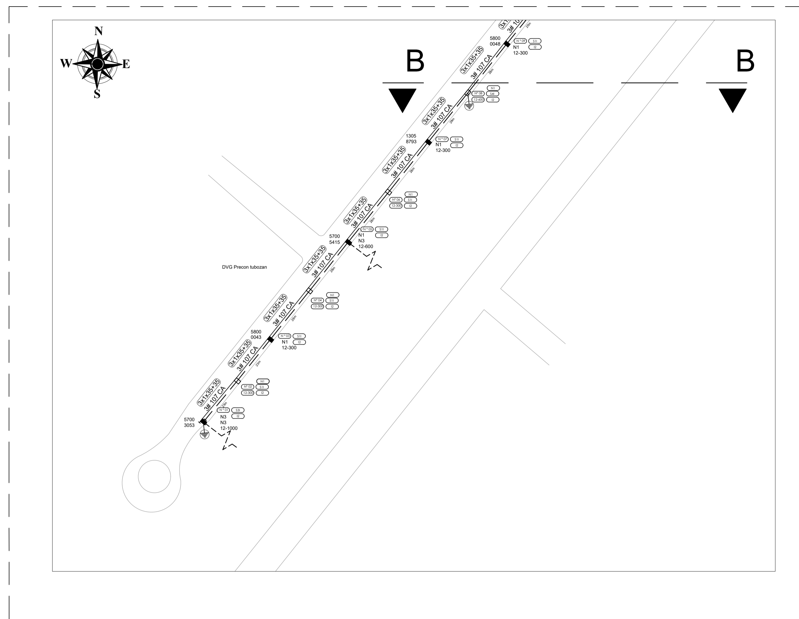
PROJEÇÃO DE ILUMINAÇÃO PÚBLICA CORTE ESCALA _____ 1:1000
