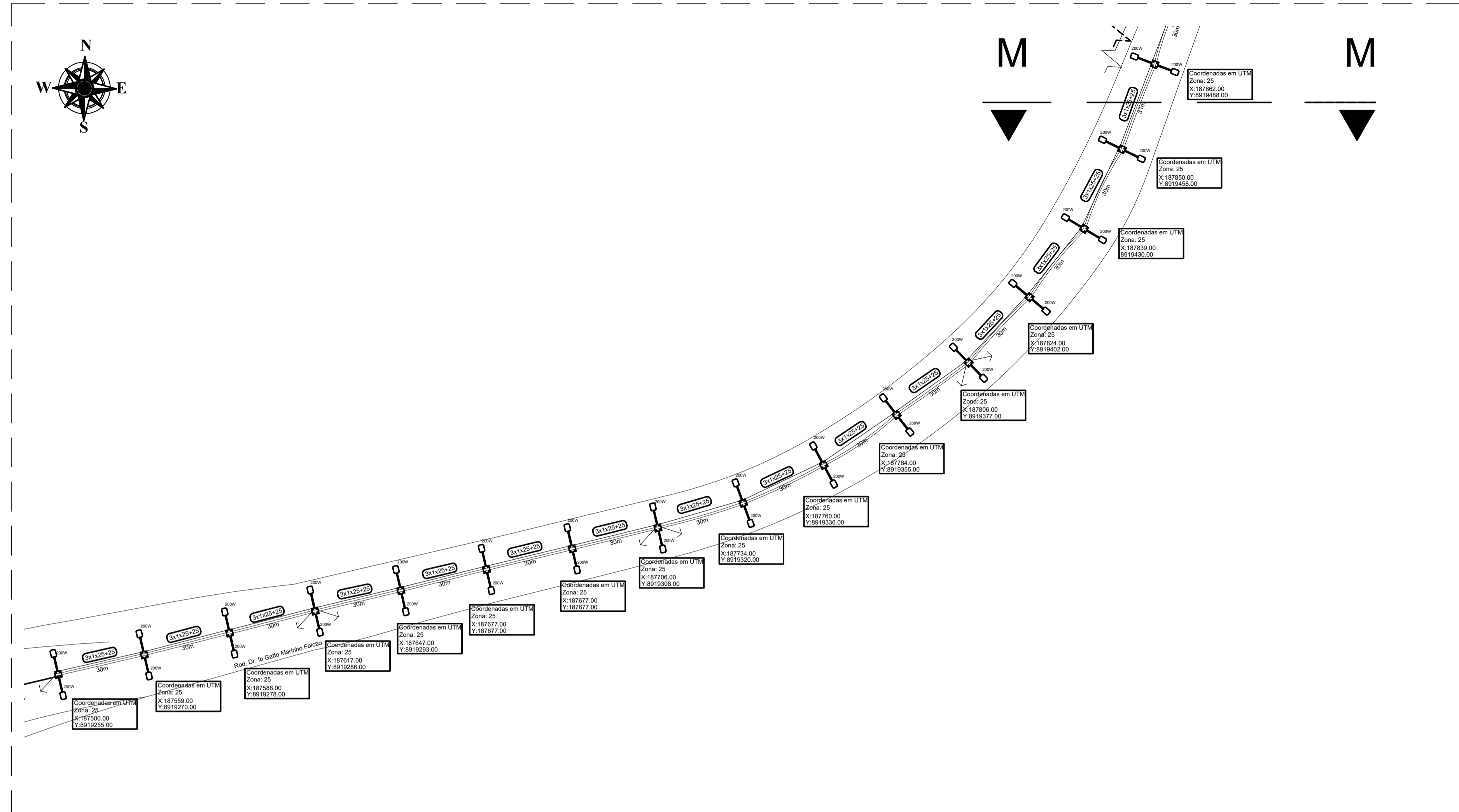
PROJEÇÃO DE ILUMINAÇÃO PÚBLICA CORTE M ESCALA 1:1000
