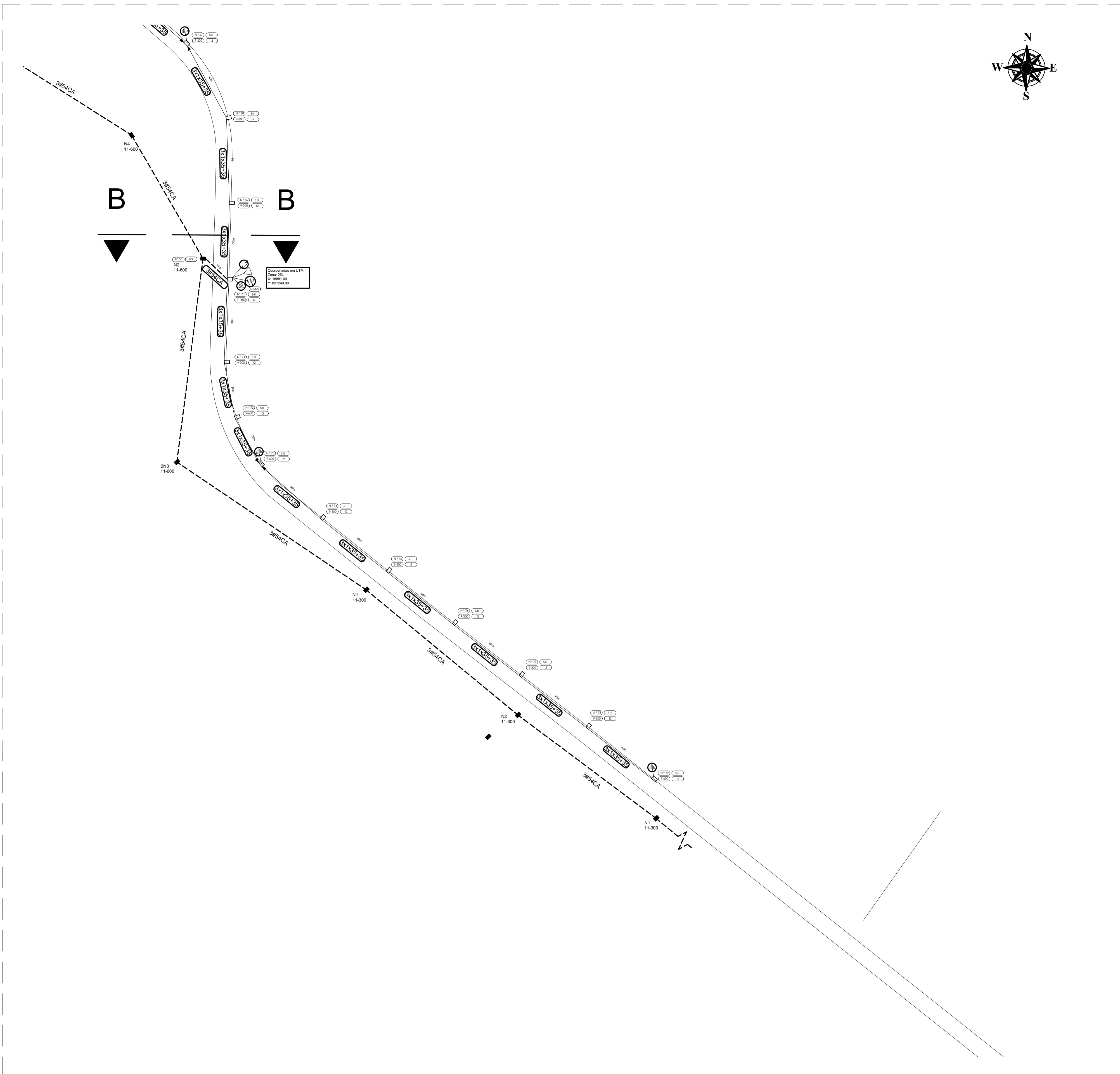
PROJEÇÃO DE ILUMINAÇÃO PÚBLICA CORTE B ESCALA _____ 1:1000
